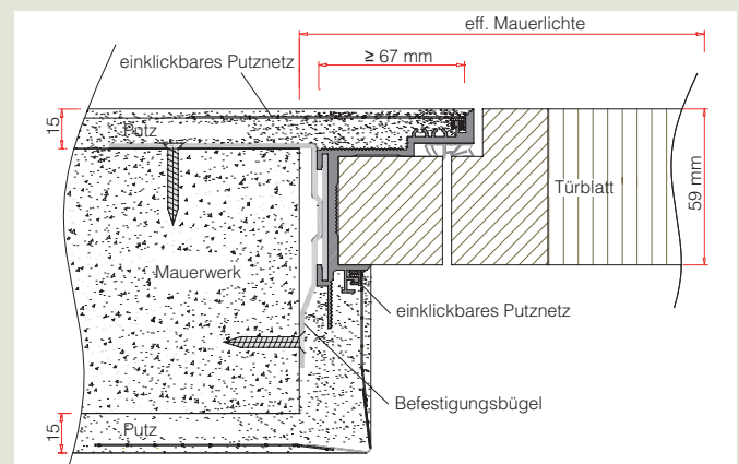
Modell TUS 59 - Türdicke 59 mm
