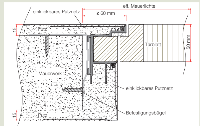
Modell TUS 50 - Türdicke 50 mm
