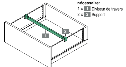
58.270.01-03 avec support 58.270.91-93 sur tube rectangulaire
