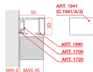
21.465.45-46 mit Profil Typ 1700/1720/1890
