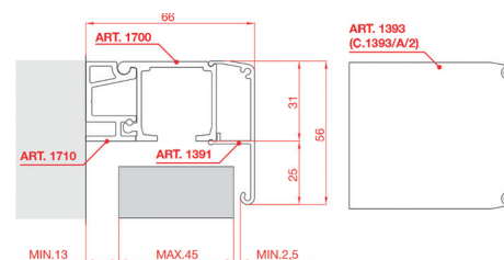
21.465.10-11 mit Profil Typ 1700/1710/1391
