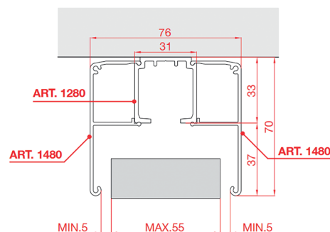
21.460.10-61 mit Laufschiene Typ 1280
