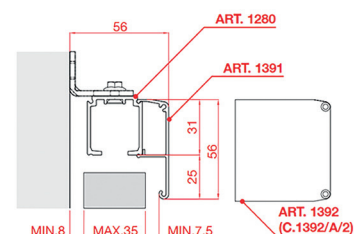
21.465.05-06 mit Profil Typ 1280/1391
