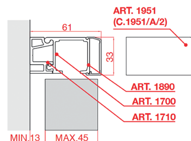
21.465.50-51 mit Profil Typ 1700/1710/1890
