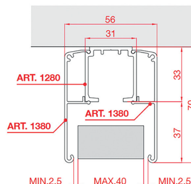
21.460.00-51 mit Laufschiene Typ 1280
