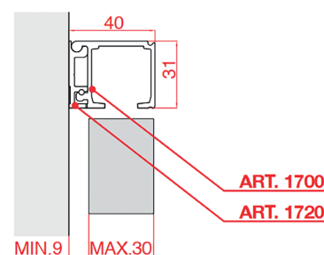
21.454.02-86 mit Profil 1720/1727
