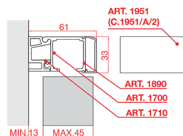
21.453.02-86 mit Profil Typ 1700/1951
