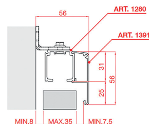
21.460.20-71 mit Laufschiene Typ 1280
