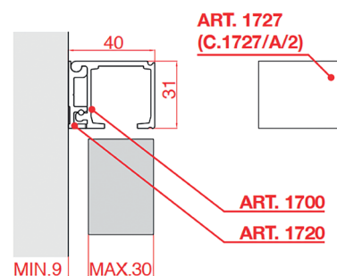
21.465.35-36 mit Profil Typ 1700/1720
