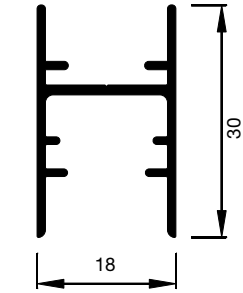
A5.6017 H-Profil
