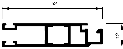
A1.3000 1252ST
