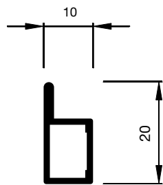
A1.3003 p-Schiene
