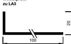
Winkelprofil zu LA3
