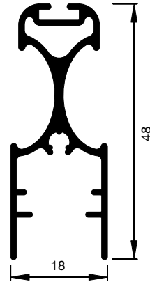
A5.6001 Griffprofil
