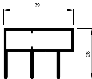
A1.3008 W-Schiene
