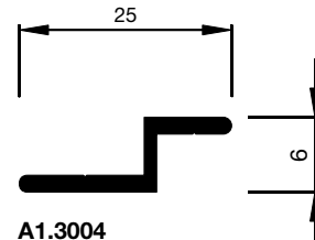
A1.3004 z-Schiene
