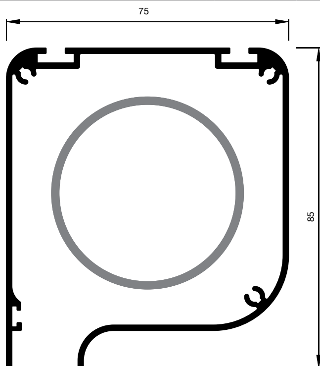
A5.5028 Kasten
