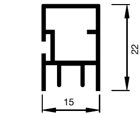
A5.6004 Frontmontageprofil
