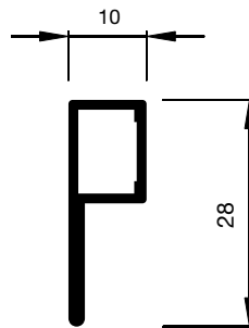
A1.3002 P-Schiene
