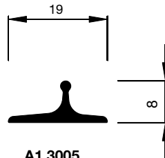
A1.3005 t-Schiene
