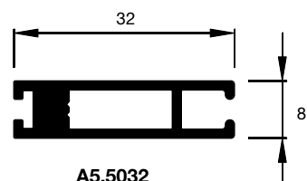
A5.5032 Zugschiene
