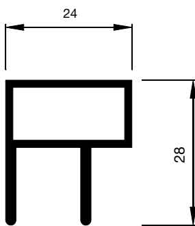
A1.3006 U-Schiene
