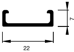
A5.6003 Bodenprofil
