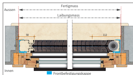
Version 3 Frontbefestigung Laibung
