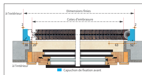
Version 4 Fixation avant
