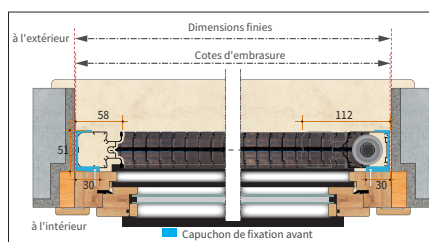
Version 3 Fixation frontale de l'embrasure
